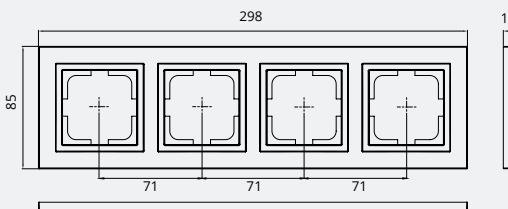
4 Gang Frame / Рамка 4-я
