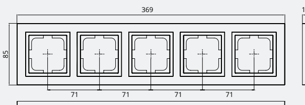
5 Gang Frame / Рамка 5-я
