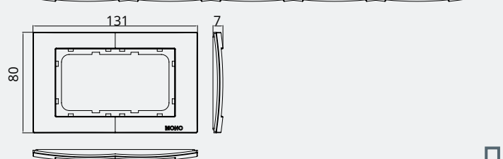
Frame for Double Socket / Двойная рамка для розетки
