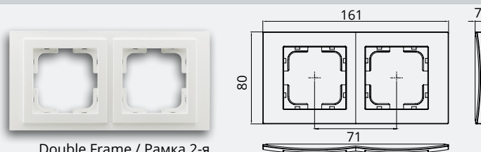
Double Frame / Рамка 2-я
