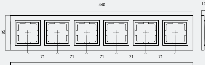
6 Gang Frame / Рамка 6-я
