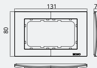
Frame for Double Socket / Двойная рамка для розетки
