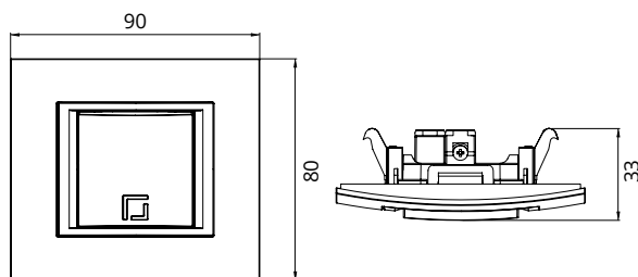
Switch Technical Drawing Технические Чертежи Выключателя
