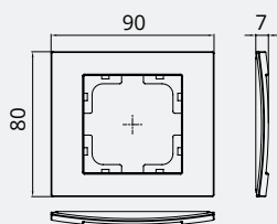
Single Frame / Рамка 1-я
