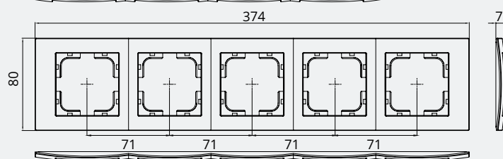
5 Gang Frame / Рамка 5-я
