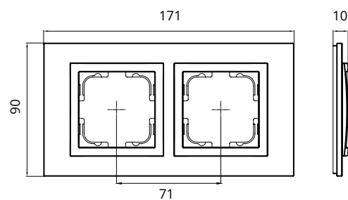
Double Frame / Рамка 2-я
