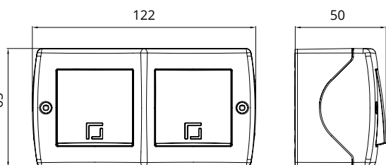
One Way Switch+One Way Switch Выключатель одноклавишный+ Выключатель одноклавишный
