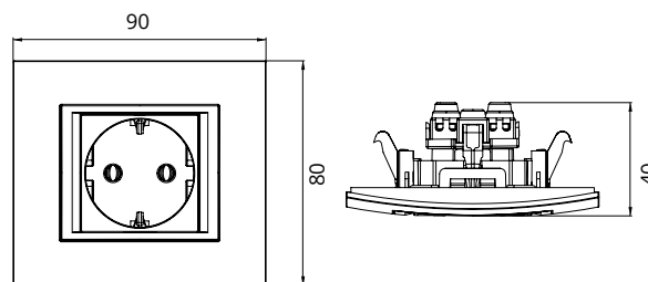
Socket Outlet Earthed Technical Drawings Технические Чертежи Розетки с Заземлением
