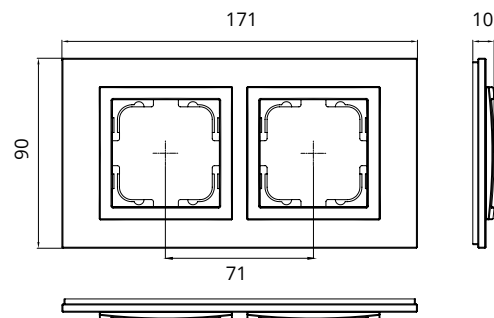
Double Frame / Рамка 2-я
