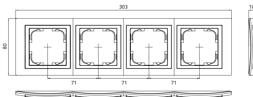
4 Gang Frame / Рамка 4-я
