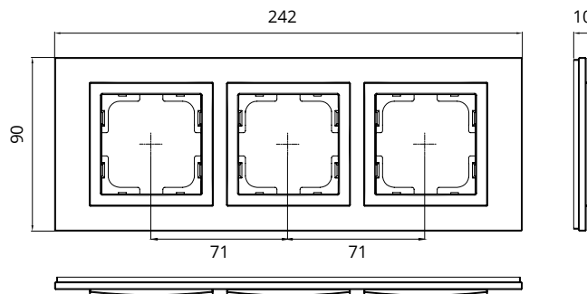
Triple Frame / Рамка 3-я
