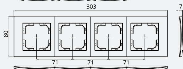
4 Gang Frame / Рамка 4-я
