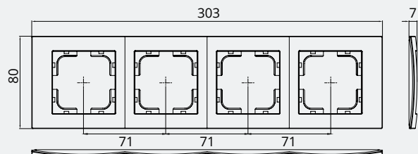
4 Gang Frame / Рамка 4-я
