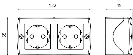
Socket Outlet Earthed+Socket Outlet Earthed Розетка с заземлением+Розетка с заземлением
