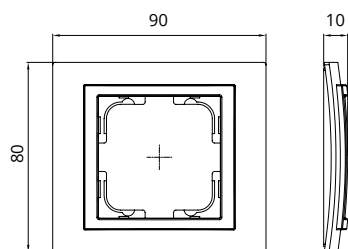
Single Frame / Рамка 1-я
