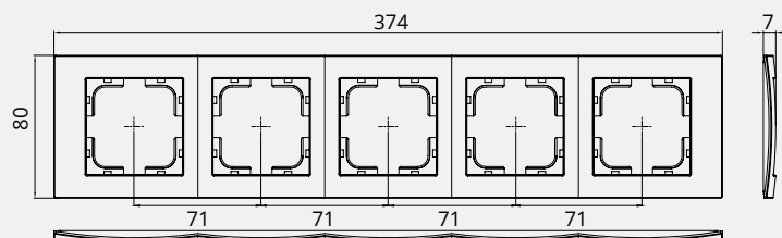
5 Gang Frame / Рамка 5-я
