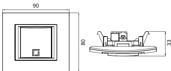
Switch Technical Drawings Технические Чертежи Выключателя
