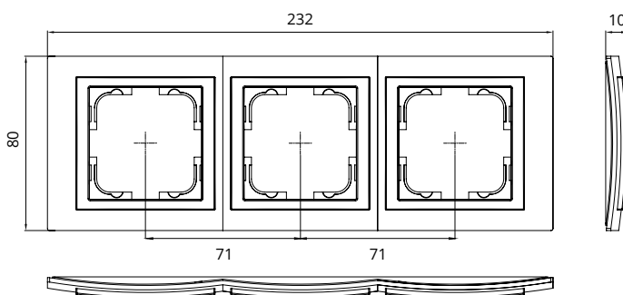
Triple Frame / Рамка 3-я
