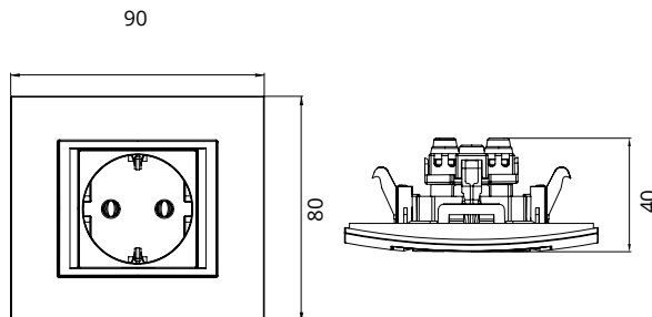
Socket Outlet Earthed Technical Drawings Технические Чертежи Розетки с Заземлением
