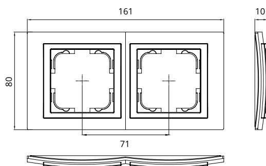
Double Frame / Рамка 2-я
