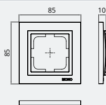
Single Frame / Рамка 1-я
