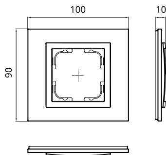
Single Frame / Рамка 1-я
