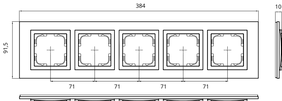
5 Gang Frame / Рамка 5-я
