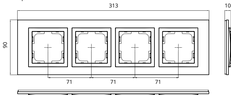
4 Gang Frame / Рамка 4-я
