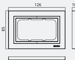
Frame for Double Socket / Двойная рамка для розетки
