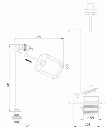
Чертеж модели 3001-I-3/8
