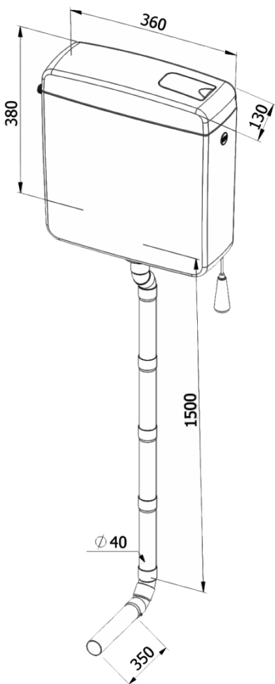
Чертеж модели 3021, 3022
