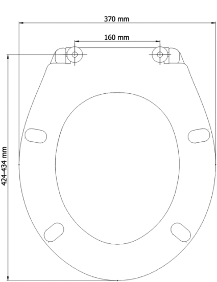
Чертеж модели 3500
