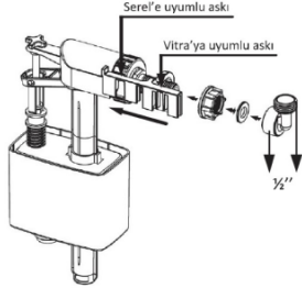
3027G-100-ASKI (в коробке) стандарт подводки шланга 3/8 дюйм латунный фитинг
