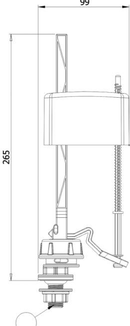
Чертеж модели 3009
