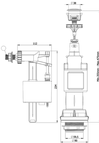
Чертеж модели 3017
