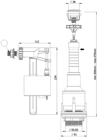
Чертеж моделей 3025
