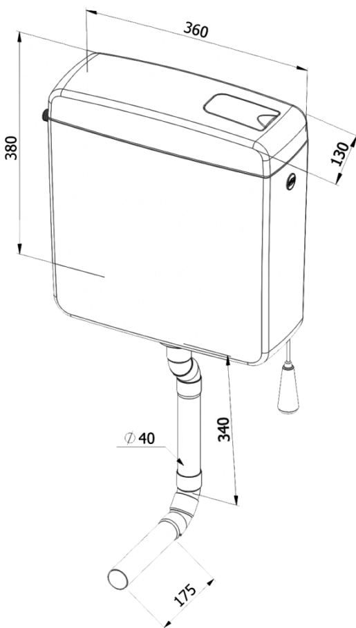
Чертеж модели 3023, 3024
