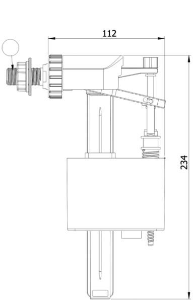
3027G-1/2-ASKI (в коробке) стандарт подводки шланга 1/2 дюйм пластиковый фитинг
