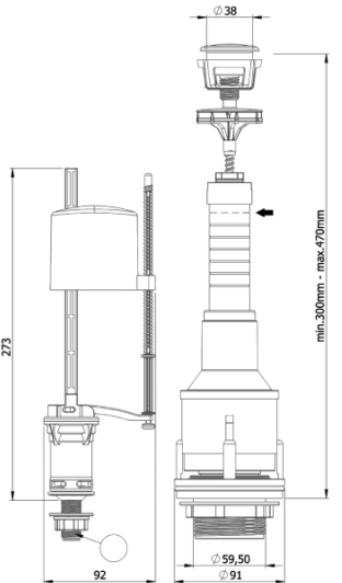
Чертеж моделей 3004
