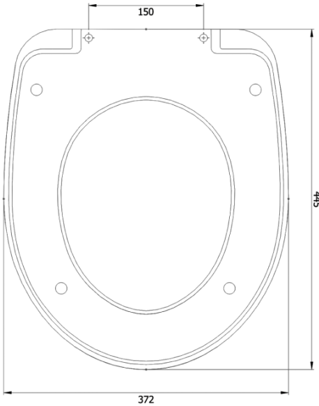
Чертеж модели 3501
