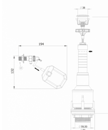
Чертеж модели 3006-I-3/8
