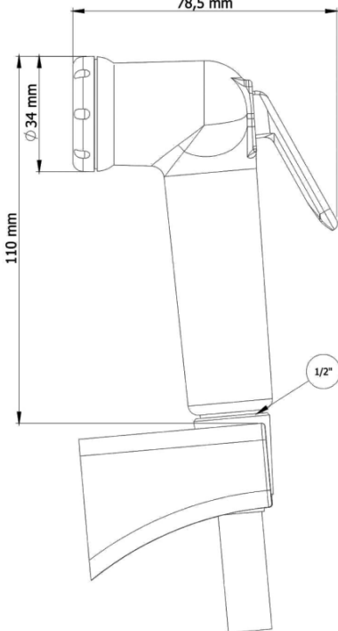
Чертеж модели 3034
