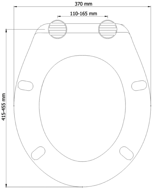
Чертеж модели 3062
