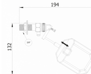
Чертеж модели 3012-I-3/8
