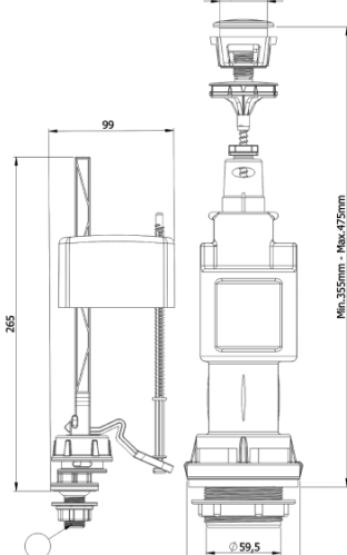
Чертеж модели 3008
