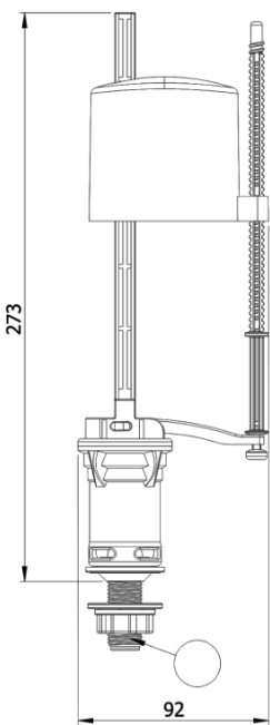
Чертеж модели 3011
