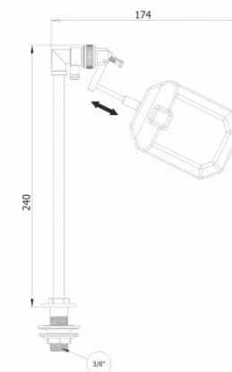
Чертеж модели 3010-I-3/8
