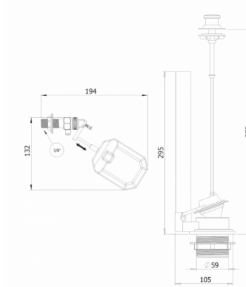
Чертеж модели 3005-I-3/8
