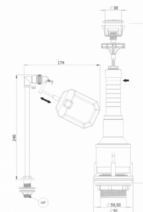
Чертеж модели 3002-I-3/8
